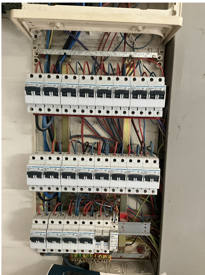
Verdeelbord 1
